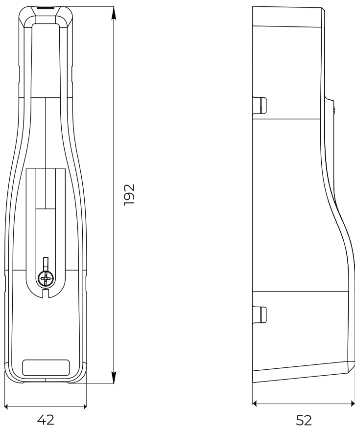
Рисунок 1 - Габаритные и установочные размеры
